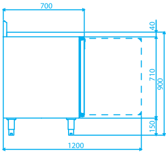
Tampo superior de encosto
